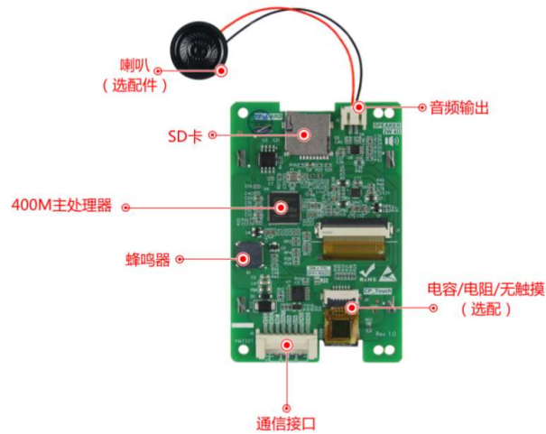
图 1-2 硬件配置图
