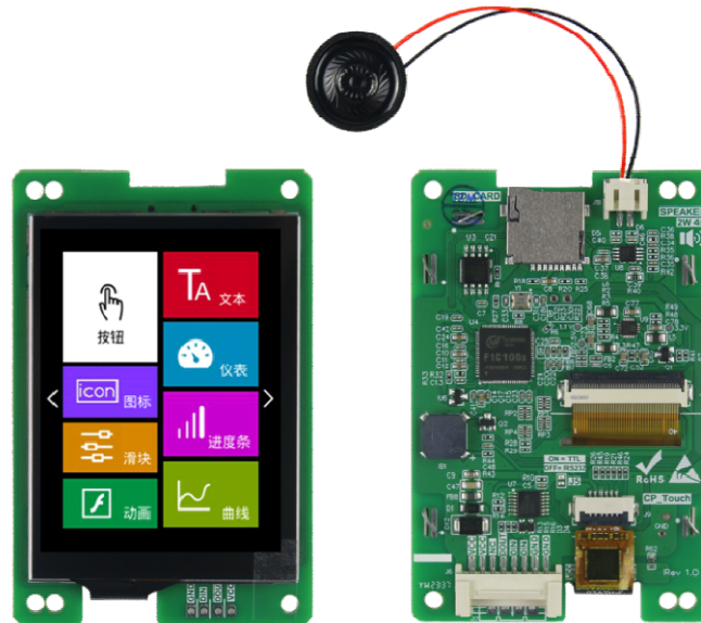
图 1-1 2.8 寸电容触摸参考图
