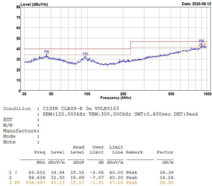
图 4-6 RE 测试垂直方向
