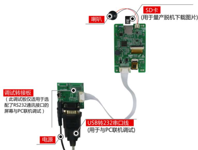
图 1-3 调试工具图
